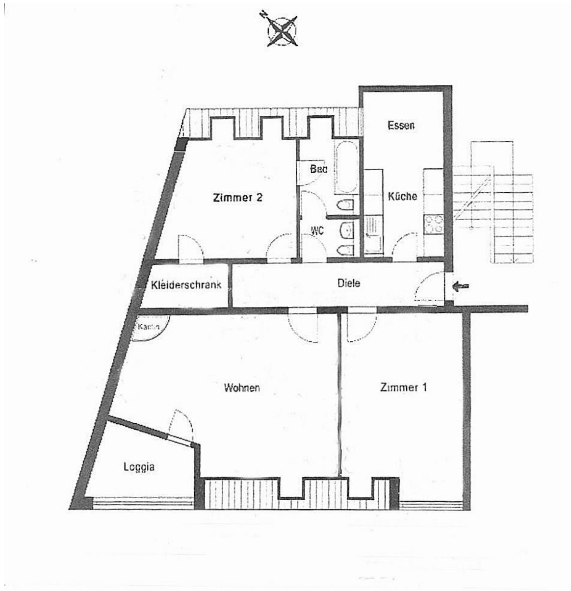
Grundriss
